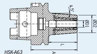
HSK-A63
