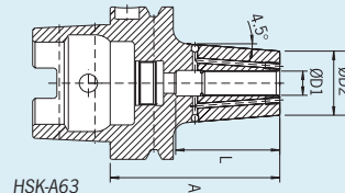
HSK-A63
