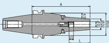
BT40
